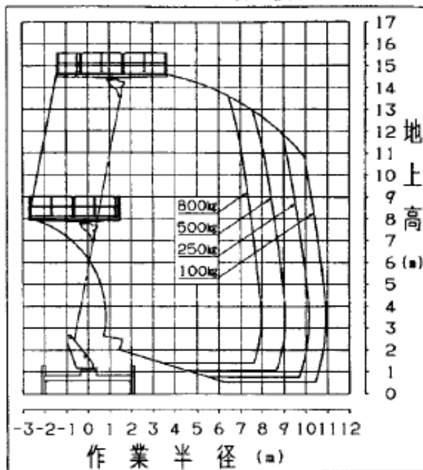
アウトリガ最大張出
